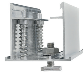
Einfache Befestigung mittels Hammerkopfschraube.
