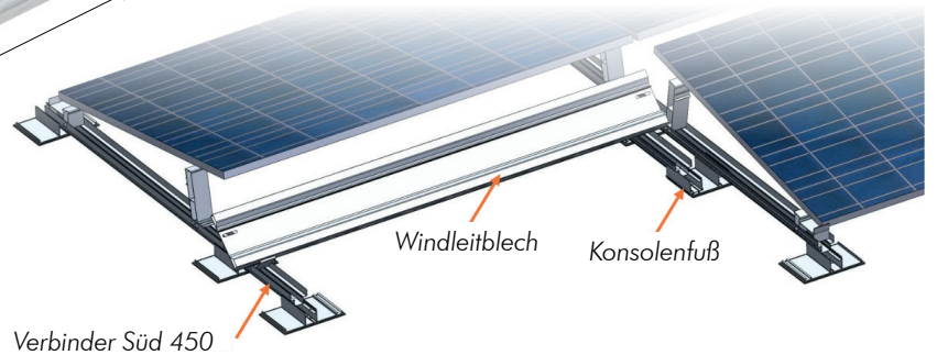
Einfache Befestigung mittels Hammerkopfschraube.
